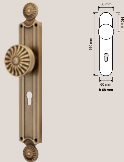
1070 FP Pomolo fisso con placca / Fixed knob on plate
