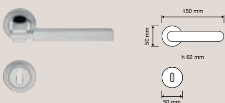
1050 RB 102 Maniglia con rosetta art.102 / Door handle on rose art.102
