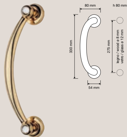
991 MN 275 108 Maniglione con rosette art.108 / Pull handle on roses art.108
