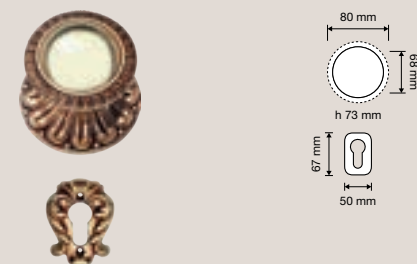
1540 PG Pomolo a girare con rosone art.1540 / Turnable knob on big rose art.1540
