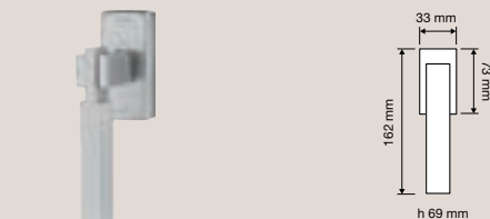
1050 SK Maniglia per finestra con movimento DK SmartBlock / Window handle with DK SmartBlock movement
