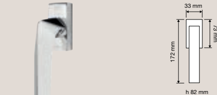
1420 SK Maniglia per finestra con movimento DK SmartBlock / Window handle with DK SmartBlock movement
